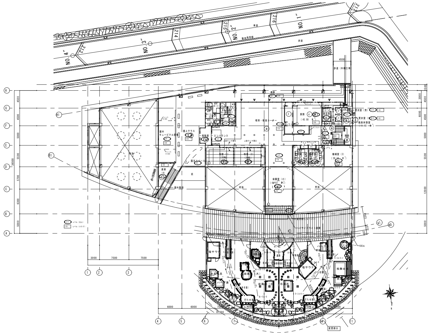
2階平面図
